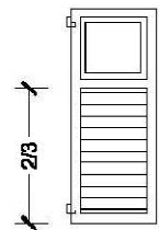
IMPOSTA IN LEGNO CON GELOSIE MOBILI MONTATE SU TELAIO FISSO
