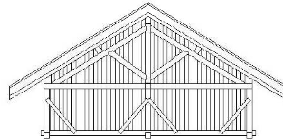
TAMPONAMENTO LIGNEO SOTTOTETTO
