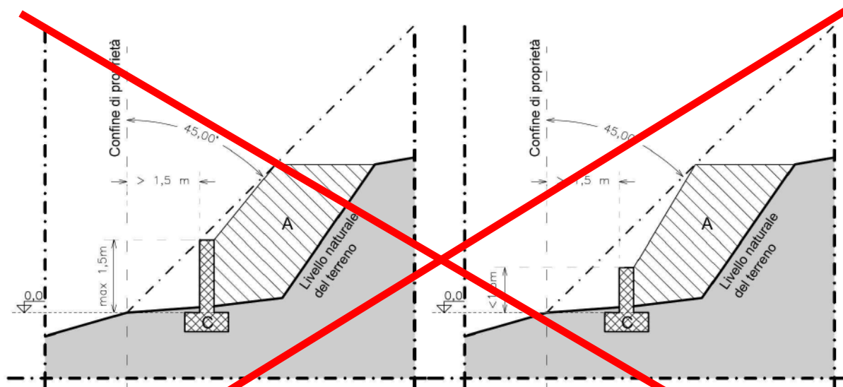
SCHEMA B.1 – distanze dei terrapieni dai confini
